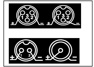
可选输出插头
